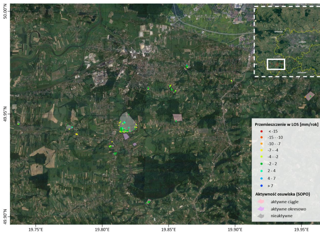
Rys. 4 Fragment obszaru badań z pomiarowymi punktami PS (orbita descending)
