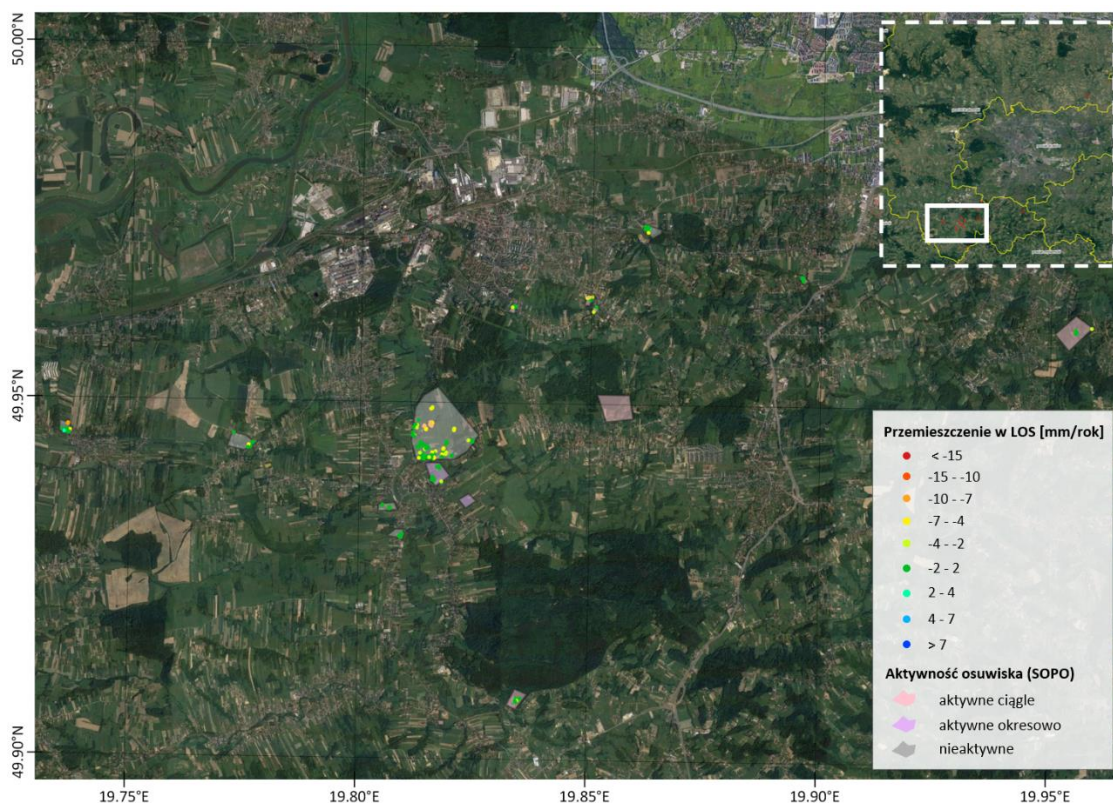
Rys. 3 Fragment obszaru badań z pomiarowymi punktami PS (orbita ascending)
