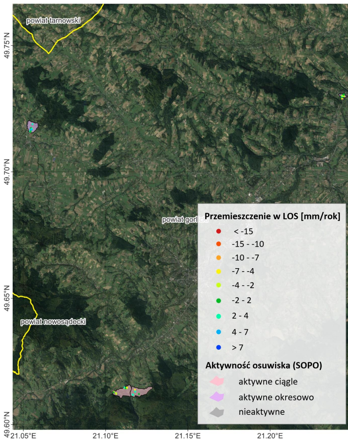
Rys. 3 Fragment obszaru badań z pomiarowymi punktami PS (orbita ascending)
