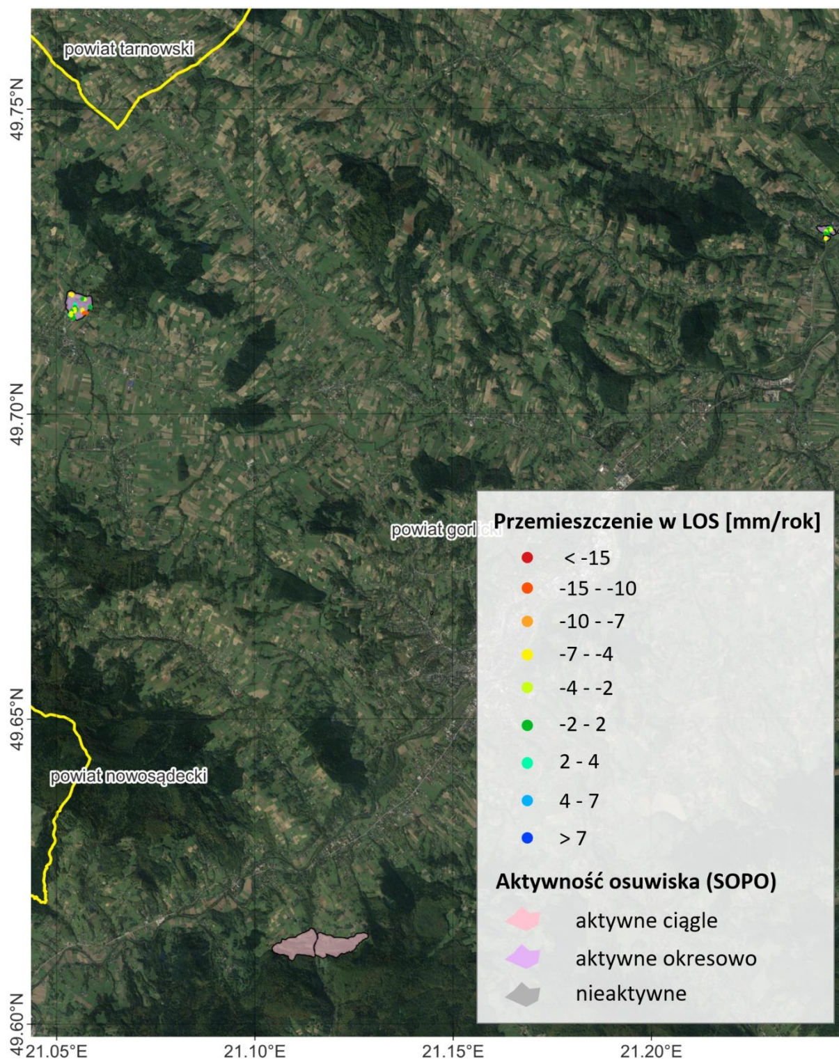
Rys. 4 Fragment obszaru badań z pomiarowymi punktami PS (orbita descending)
