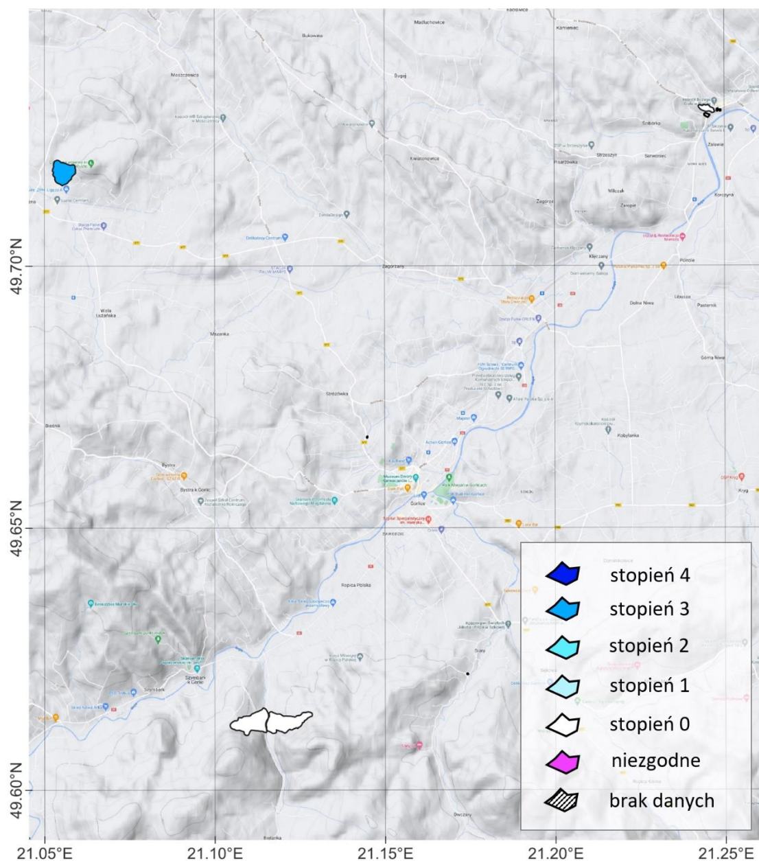
Rys. 7 Mapa intensywności ruchów osuwisk (fragment)
