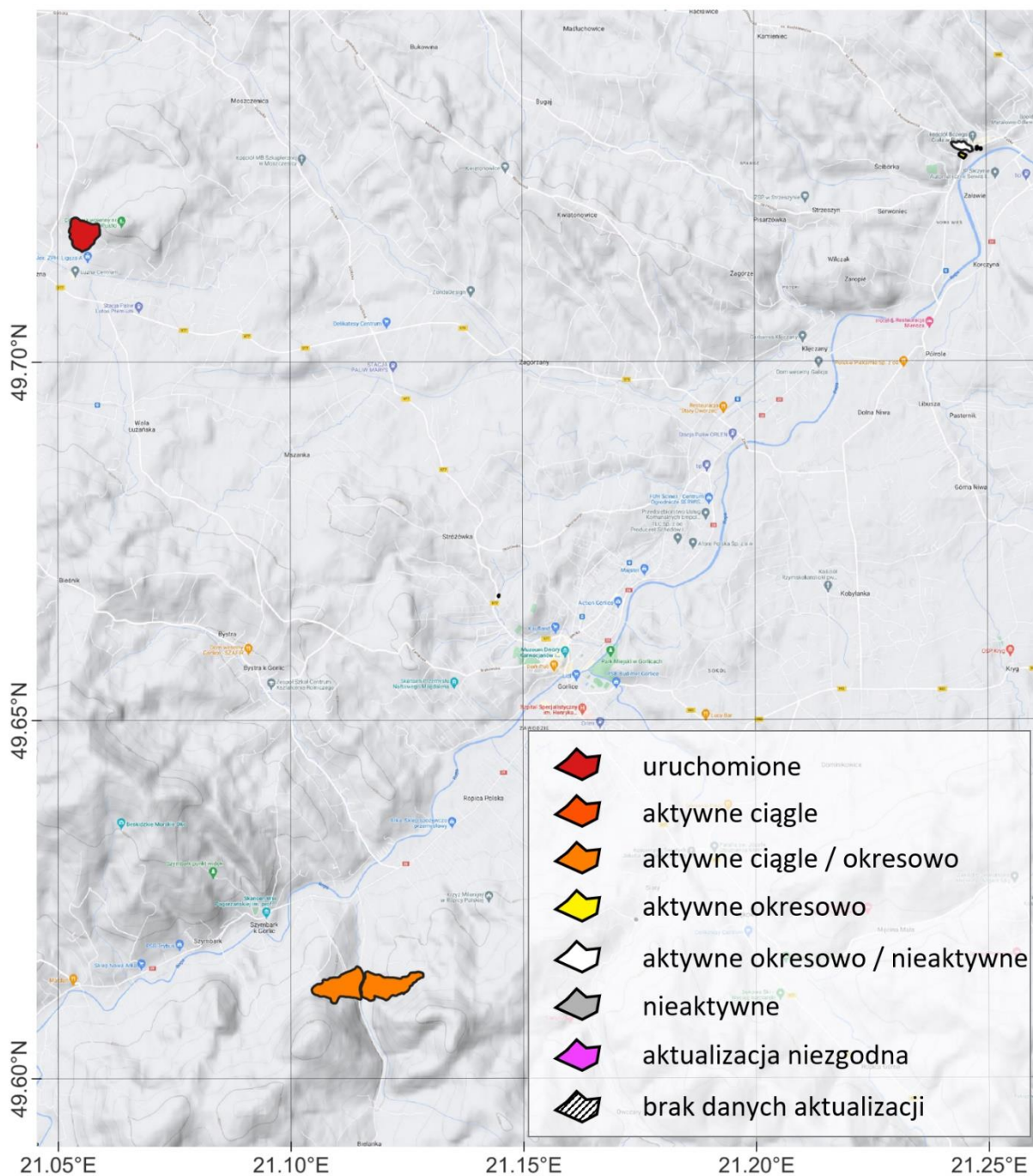
Rys. 6 Mapa zaktualizowanej aktywności osuwisk (fragment)
