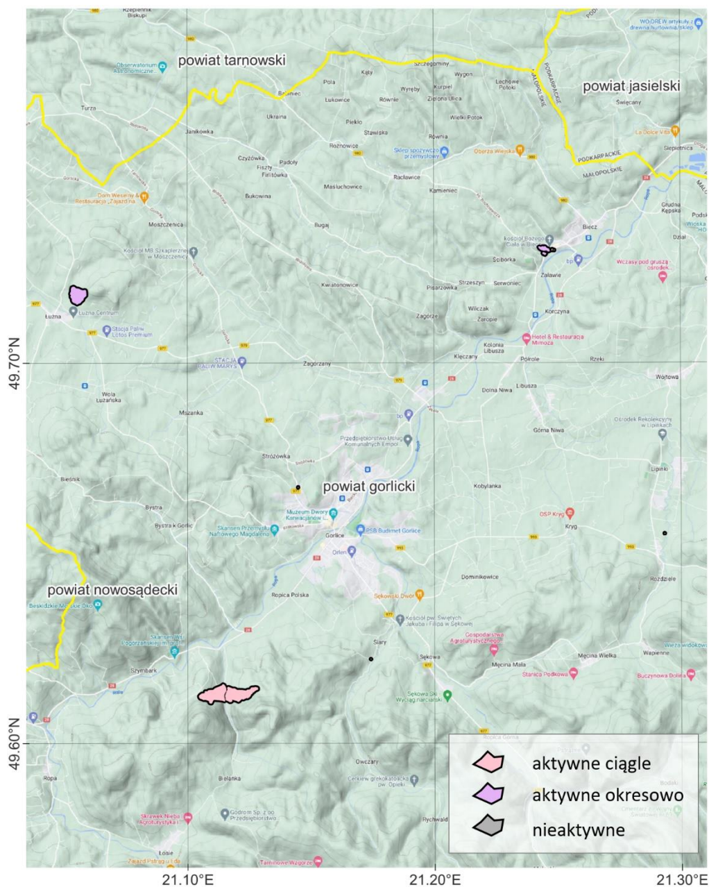
Rys. 1. Obszar badań z granicami osuwisk SOPO
