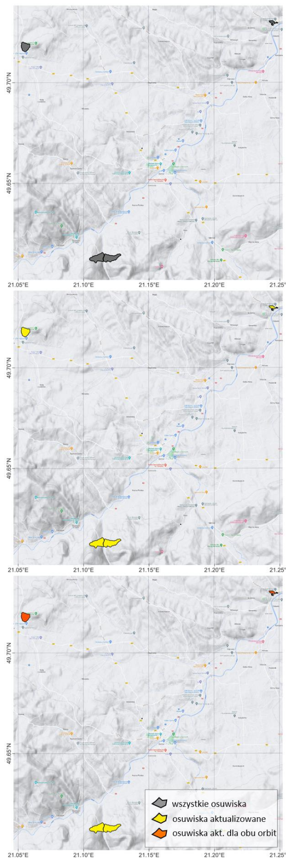
Rys. 5 Mapa selekcji osuwisk
